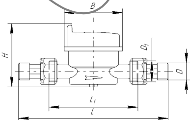
Рисунок 1 – схематическое изображение счетчика.
